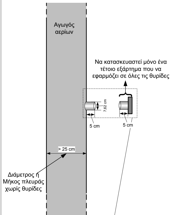
Σχέδιο 3β: Θυρίδα/ες για μετρήσεις σκόνης και αερίων για κυκλικά φουγάρα με διάμετρο που υπερβαίνει τα 25 cm και ορθογώνια / τετράγωνα φουγάρα που το μήκος της πλευράς χωρίς θυρίδες υπερβαίνει τα 25 cm
