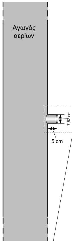
Σχέδιο 3α: Θυρίδα/ες για μετρήσεις σκόνης ανεξάρτητα από τις διαστάσεις φουγάρου
