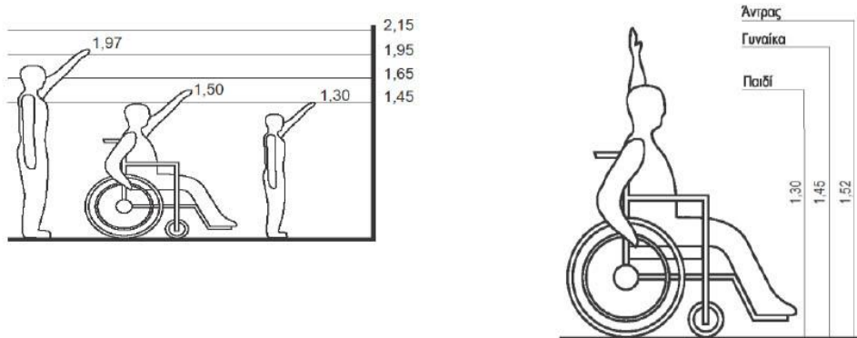
Σχήμα 4: Ανθρωπομετρικές διαστάσεις.
