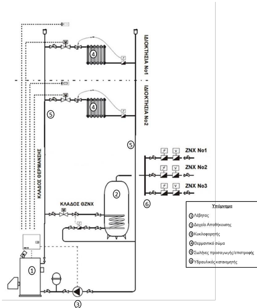
Εικόνα 2: Εγκατάσταση κεντρικού συστήματος παραγωγής ζεστού νερού οικιακής χρήσης σε σύνδεση με το σύστημα κεντρικής θέρμανσης
