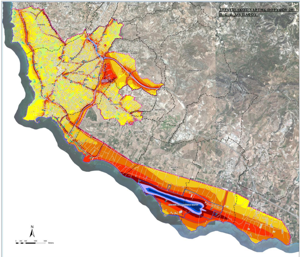
Στρατηγικός Χάρτης Θορύβου Πολεοδομικού Συγκροτήματος Πάφου – Δείκτης Lden (24 ώρες) Συνδυασμένος Περιβαλλοντικός Θόρυβος (οδικός, αεροπορικός και βιομηχανικός)
