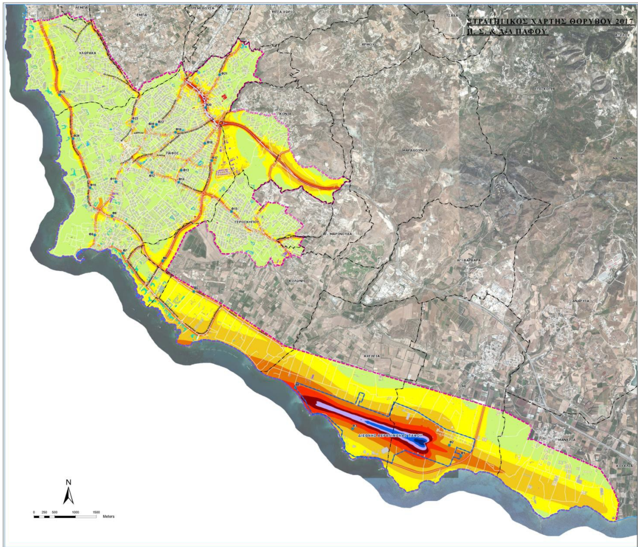
Στρατηγικός Χάρτης Θορύβου Πολεοδομικού Συγκροτήματος Πάφου – Δείκτης L_{night} (23:00-07:00) Συνδυασμένος Περιβαλλοντικός Θόρυβος (οδικός, αεροπορικός και βιομηχανικός)
