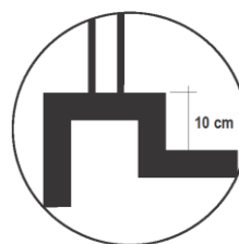
Σχήμα 36- Προστατευτικό περίζωμα εκατέρωθεν της ράμπας, ύψους 0,10μ.
