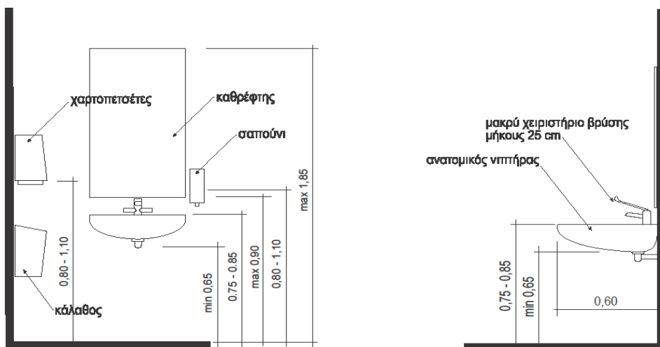
Σχήμα 86 - Νιπτήρας σε πλάγια όψη. Η αποχέτευση του νιπτήρα δεν πρέπει να εμποδίζει τα γόνατα του χρήστη.
