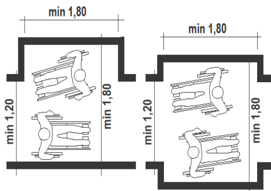
Σχήμα 28-. Διαπλάτυνση 1,80X1,80 μ. τοπικά σε διαδρομή πλάτους 1,20 μ.
