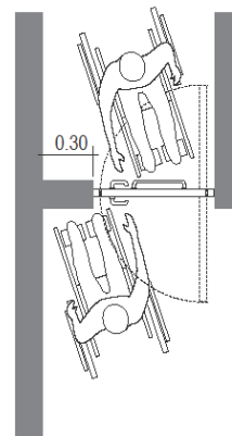
Σχήμα 59- Θύρα με ελεύθερη απόσταση 0,30μ από τον τοίχο σε πολυκατοικίες με γραφεία και σε εισόδους γραφείων.
