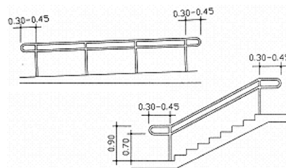
Σχήμα 47- Διπλός χειρολισθήρας.
