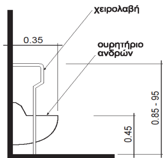
Σχήμα 74- Ουρητήρας χρήστη τροχοκαθίσματος.
