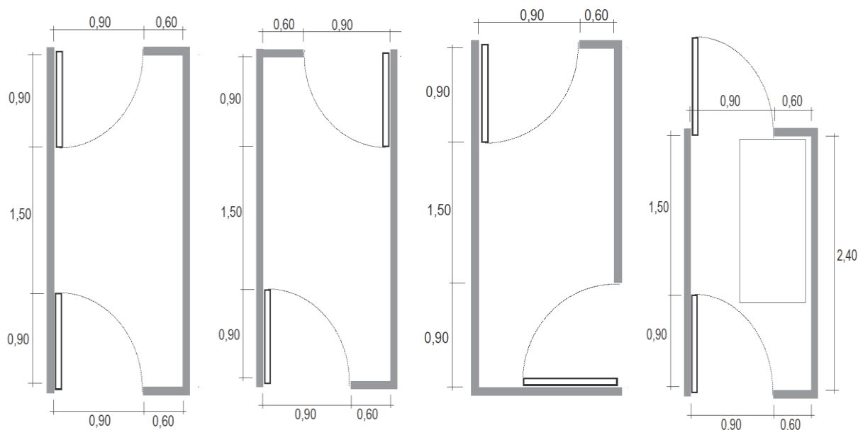
Σχήμα 63- Προθάλαμοι Παραδείγματα προθαλάμων κτηρίων με χρήση κοινού με ανεμπόδιστη απόσταση μήκους 1,50μ για τους ελιγμούς τροχοκαθίσματος.
