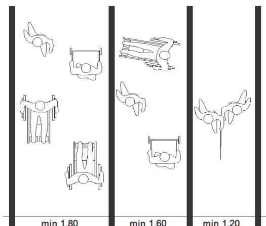
Σχήμα 27- Ελεύθερο πλάτος διαδρομών απαλλαγμένων από οποιαδήποτε εμπόδια.
