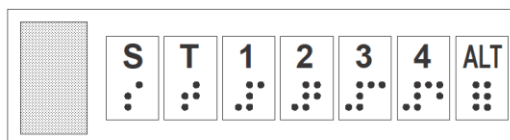
Σχήμα 66- Χειριστήρια του ανελκυστήρα σε οριζόντια τοποθέτηση, με ανάγλυφη ένδειξη σε γραφή Μπρέιλ.
