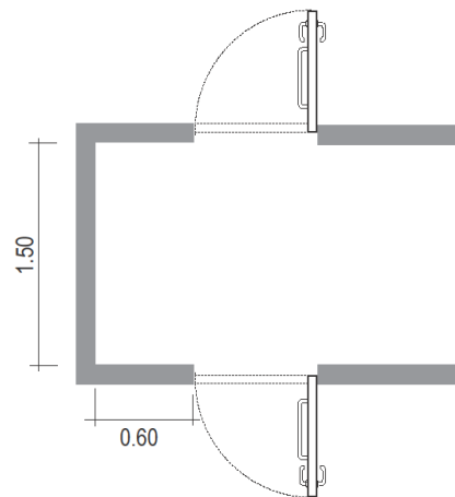
Σχήμα 62- Διάδρομος πλάτους 1,50.
