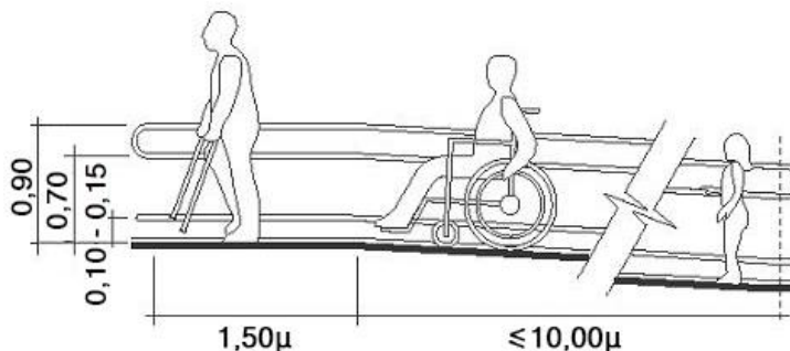
Σχήμα 37- Πλάγια όψη ράμπας
