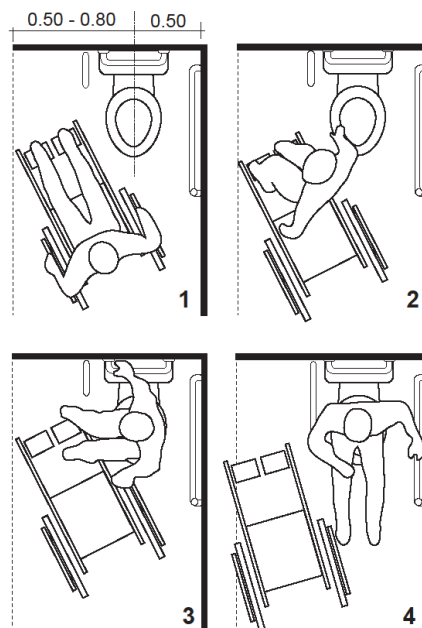
Σχήμα 73- Κάθετος τρόπος μεταφοράς
